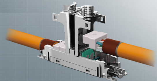
fixLink ® Extender Kat.6 A ISO/IEC CKEFFL00 (AWG 24-22) CKEFFLFL (AWG 27-26)
