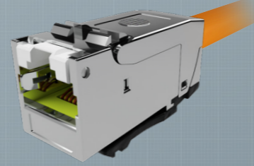
fixLink ® Pro + Keystone Kat.8.1 ISO/IEC CKFAK002P+ (AWG 26-22)
