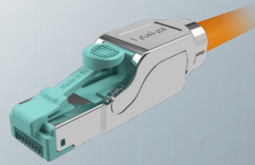
fixLink ® RJ45 Plug Kat.6 A ISO/IEC CKFFK001 (AWG 26-22)
