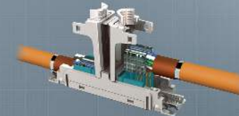
preLink ® Extender Kat. 6, ISO/IEC CKEA0100 (Solid-Variante)
