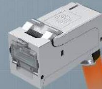
preLink ® RJ45 Keystone gewinkelt Kat. 6, ISO/IEC CKWAS011 (Solid-Variante) CKWAS021 (Flex-Variante)
